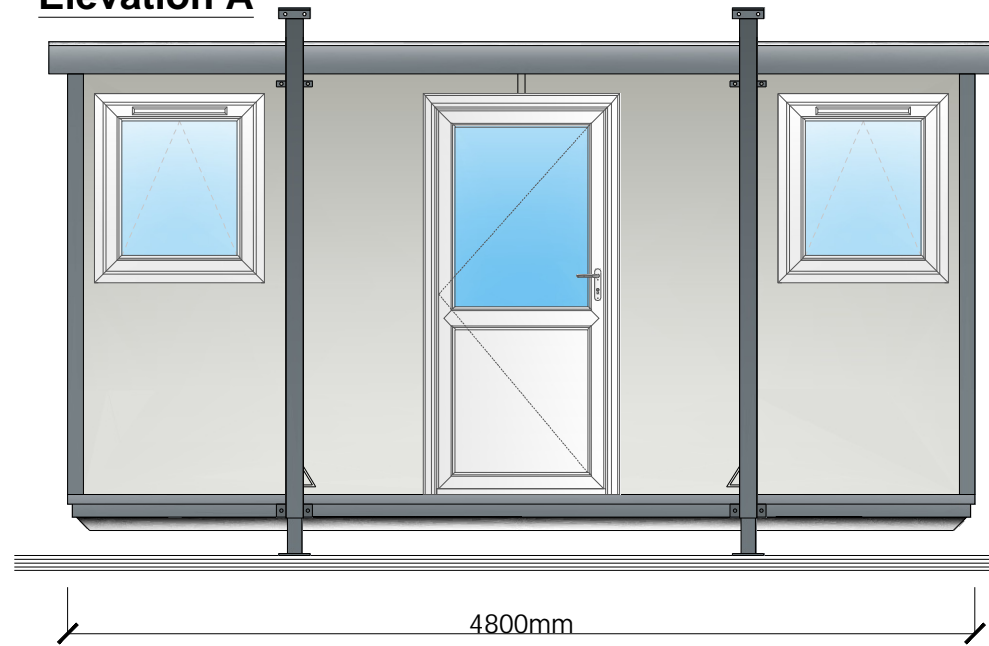
Elevation A
