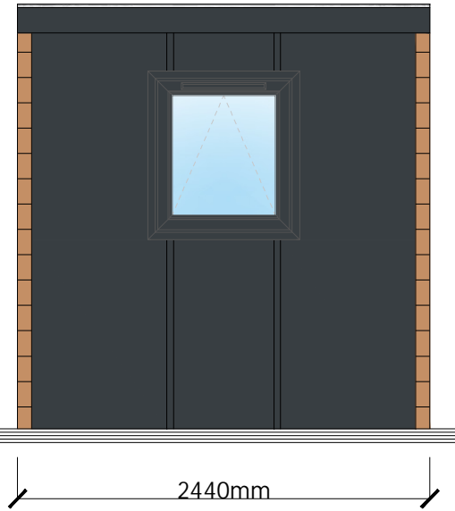
Elevation B
